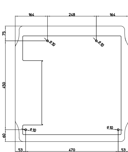
Abb. 2: rückseitige Metallplatte für die Wandmontage der Station
