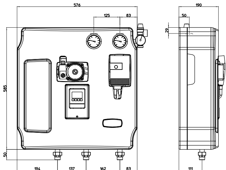
Abb. 3: wichtige Maße und Achsabstand der Station
